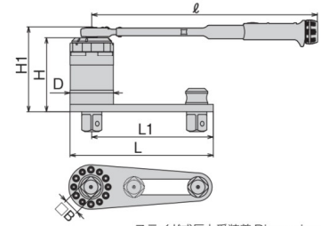
スライド式反力受装着 Dimensions 図
