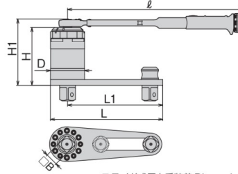
スライド式反力受装着 Dimensions 図
